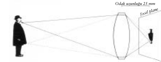
Şekil 8: Kısa odak uzunluklu bir merceğin oluşturduğu görüntü
