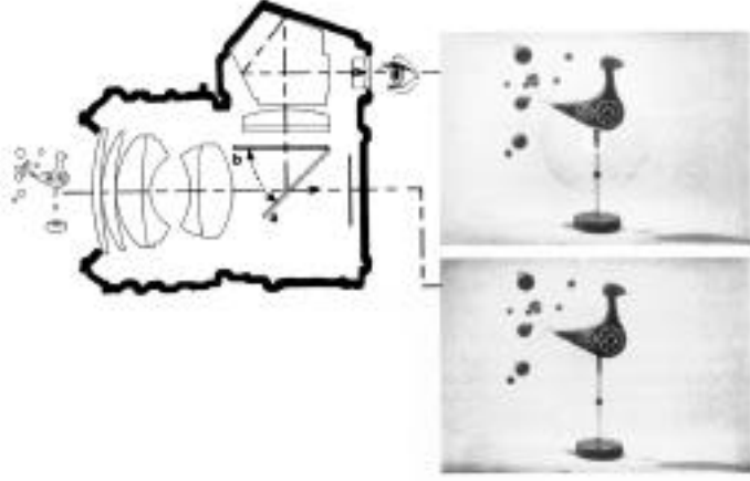
Şekil 14: SLR Fotoğraf Makinesi Şeması
