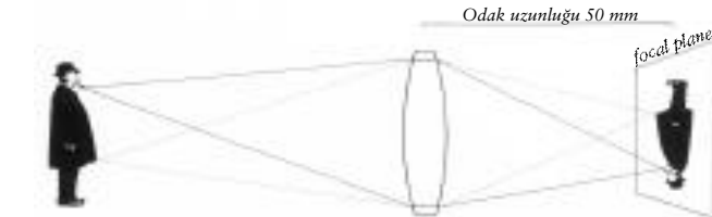
Şekil 9: Uzun odak uzunluklu bir merceğin oluşturduğu görüntü
